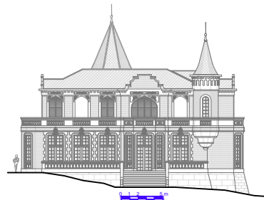
Elevação 02
