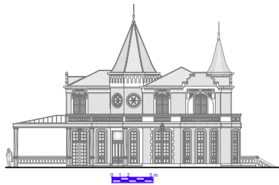
Elevação 01
